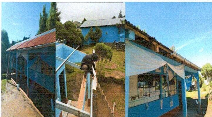
Foto 2: Estructura de techo: Sustitución de estructura de soporte de madera por metal
