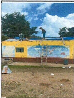
Foto1: cubierta de lamina:Sustitución de lamina troquelada calibre 26
