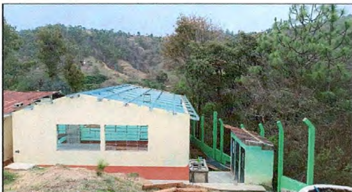
Foto 9: Sustrución de vigas y reglas de madera por costaneras y tubos de metal.
