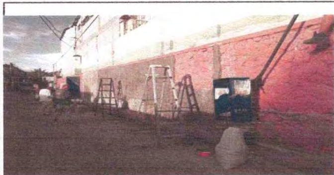
Foto 1: tres manos relleno, repello y sernido de muro perimetral de pared frontal exterior entrada y calle principal del establecimiento
