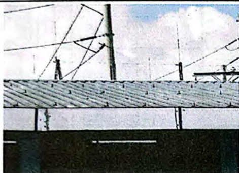
Foto 1: Suministro y aplicación de sika a tornillos de techo.
