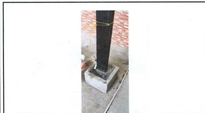
Foto 3: bases de concreto para columna techo de patio
