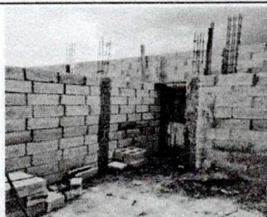
Foto 2: Fundición de las columnas frontales
