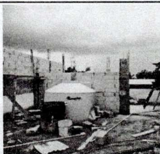
Foto 3: División construida para area del baño
