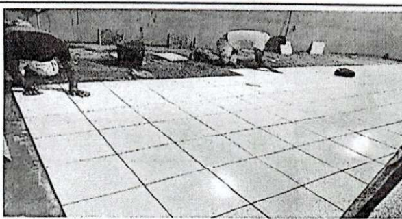
Foto 6: Instalación de piso cerámico en Salón de 1o. Básico.
