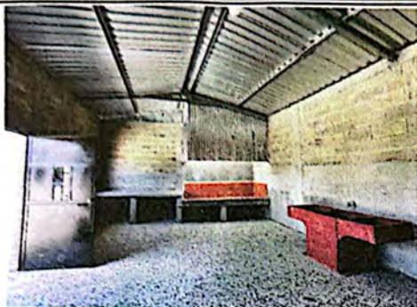
Foto 1: Muros de mampostería reforzados para ampliación de cocina.
