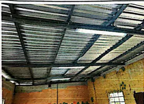
Foto 5: Colocación de estructura para techo, con aplicación de pintura anticorrosiva.
