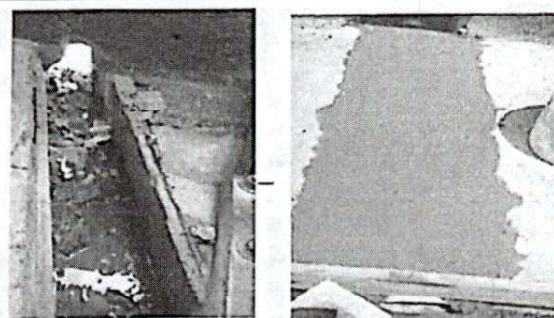
Foto 12: reparación de salida de agua pluvial interna
