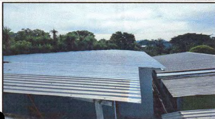
Foto1: Cubierta de lámina y estructura de techo de ambiente cocina, cambio de lámina galvanizada por lámina troquelada aluzin 13' y 14', calibre 26 legítimo sustitución de estructura de soporte de madera, por metal(costaneras)
