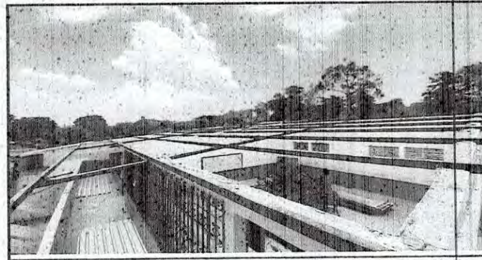
Foto 6: Sustitución de lámina galvanizada por lámina troquelada Aluzin 13' y 18', calibre 26 legítimo
