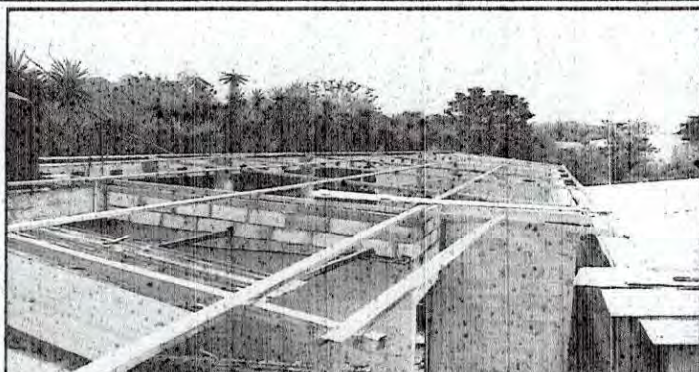
Foto 1: Cubierta de lámina y estructura de techo de ambiente cocina, cambio de lámina anizada por lámina troquelada aluzin 13' y 14', calibre 26 legítimo sustitución de estructura de soporte de madera, por metal(costaneras)
