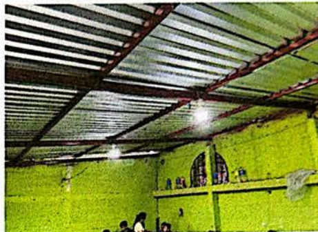
Foto 2: Suministro e instalación de lámina troquelada en salón de clases.
