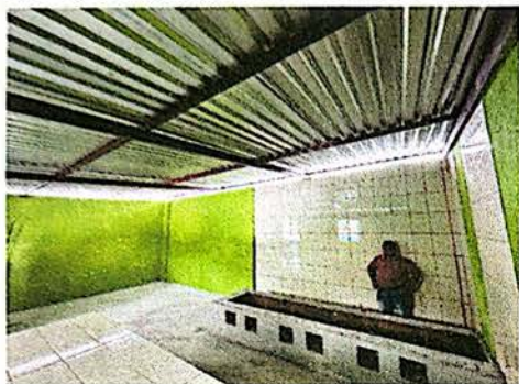
Foto 7: Suministro e instalación de estructura metálica para soporte de techo + Lámina troquelada + instalación de azulejo en muro.
