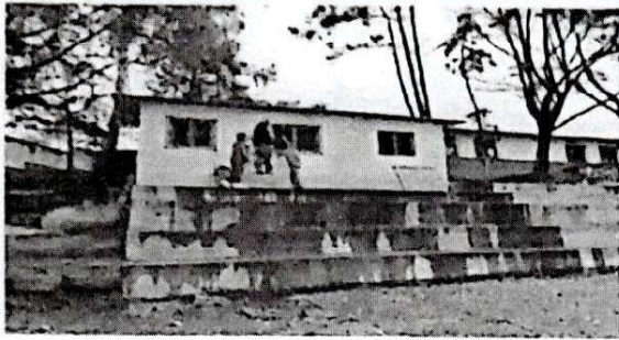
Foto 1: Proceso de cambio de techo aula 5
