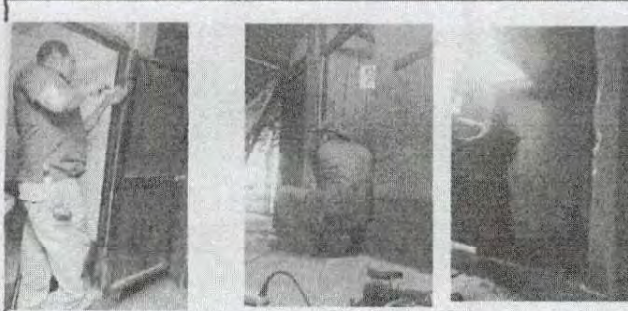
Foto 6: Desinstalando puertas de sanitarios, de madera para luego colocar puertas de metal en el segundo piso, frente a primero b.
