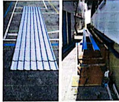
Foto 8: Estructura metálica y lámina para fabricación de cubierta en cocina.
