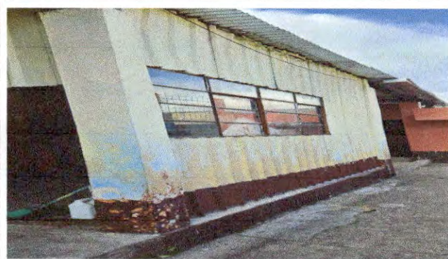
Foto 9: SUMINISTRO Y COLOCACION DE BLOCK CON REFUERZO ESTRUCTURAL
