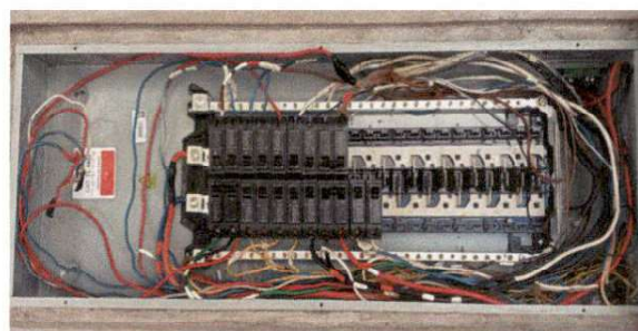
Foto 6: Sistema Eléctrico: se sustituyo la caja o tablero
