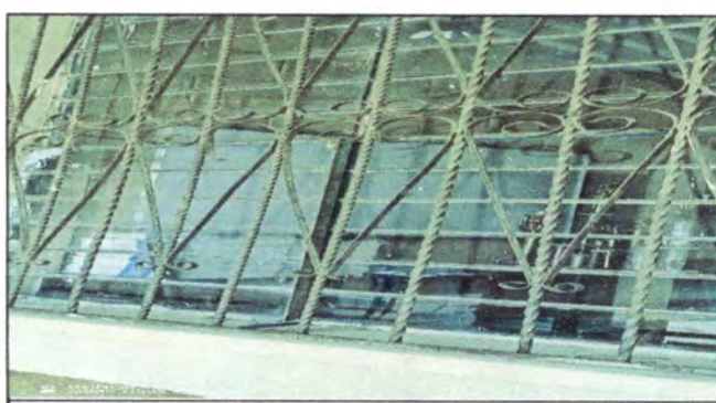
Foto 18: Mantenimiento de un balcón en la clase de segundo primaria con medida de 6 metros cuadrados y un balcón en la bodega vespertina con cuatro metros cuadrados en la planta baja. Lijado, cepillado, aplicación de pintura anticorrosiva, soldar piezas de adorno sueltas.
