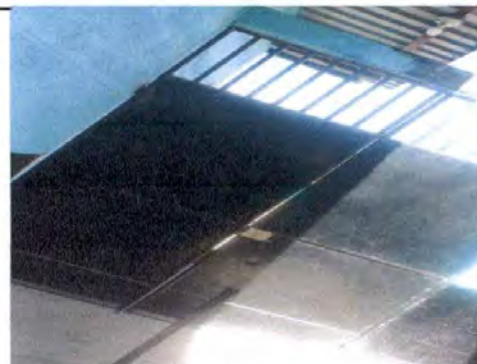
Foto 12: 12.1 Mantenimiento a porton de metal que incluye lijado, cepillado, aplicación de pintura anticorrosiva y mantenimiento de chapa.
