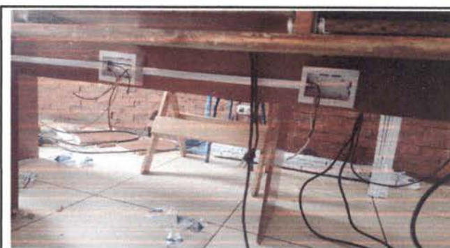
Foto 4: 19.12 Instalación de unidades de fuerza, tomacorrientes dobles en área de computación para corregir todas las instalaciones de fuerza. (Incluye sustitución de cableado y ducto eléctrico con sus respectivos accesorios)
