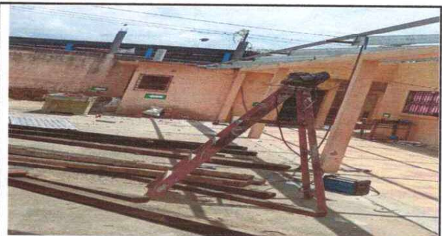
Foto 10 : Se encuentra en proceso la instalacion de pescantes para canal de aguas pluviales.
