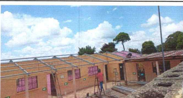
FOTO 5: Finalización de instalación de estructura de soporte de metal.
