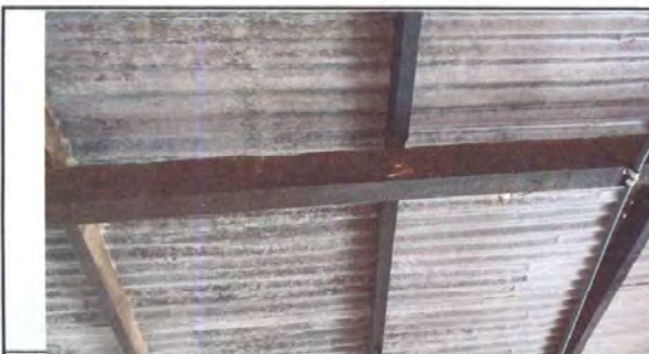
Foto 5: Sustrucción de estructura de soporte de madera, por metal por encontrarse en muy mal estado.
