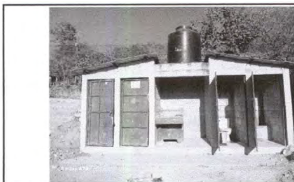
Foto 5: Cada módulo de baño tendrá azulejo (renglón 13) y el mingitorio (renglón 19.15) se cambiará por uno de porcelana. Así como sustitución de accesorios de inodoro (renglón 10.2)
