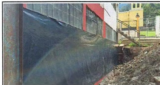
Foto 29: Muro exterior de salones, reparado.
