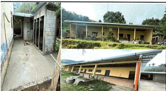
FOTO: 07-09: AREA DE MODULOS DE SALONES, CUBIERTA DE LAMINA ONDULADA, ESTRUCT. DE MADERA EN MAL ESTADO. SUSTI. POR LAMINA TROQUEL. CAL. 26 Y ESTRUCT. METALICA
