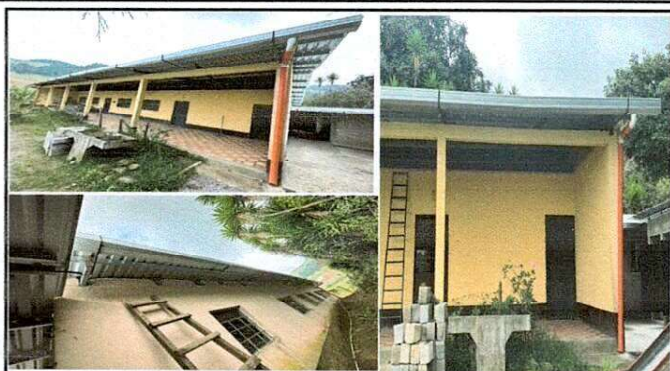
FOTO: 04-06: AREA DE MODULO DE SALONES, CUBIERTA DE LAMINA ONDULADA, ESTRUCT. DE MADERA EN MAL ESTADO. SUSTI. POR LAMINA TROQUEL. CAL. 26 Y ESTRUCT. METALICA
