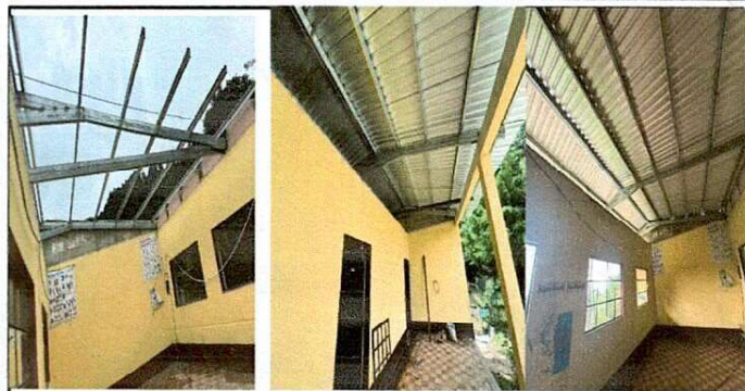
FOTO: 04, 05 Y 06 AREA DE MODULOS DE SALONES, CUBIERTA DE LAMINA ONDULADA A SUSTITUIR, Y ESTRUCTURA DE MADERA EN MAL ESTADO, POR LAMINA TROQUELADA NUEVA CAL. 26 Y ESTRUCTURA METALICA.
