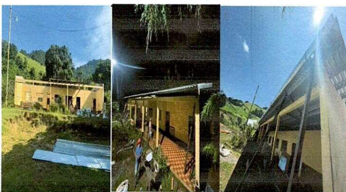
FOTO: 07, 08 Y 09 MODULO DE SALONES Y CORREDOR, CUBIERTA DE LAMINA ONDULADA A SUSTITUIR, Y ESTRUCTURA DE MADERA EN MAL ESTADO, POR LAMINA TROQUELADA CALIBRE 26Y EST. METALICA
