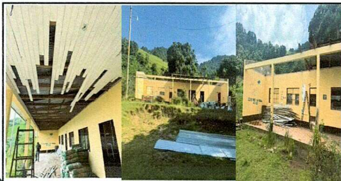
FOTO: 01, 02 Y 03 AREA DE MODULOS DE SALONES, CUBIERTA DE LAMINA ONDULADA, A SUSTITUIR, ESTRUCTURA DE MADERA, POR LAMINA TROQUELADA NUEVA CAL. 26 Y ESTRUCTURA METALICA.
