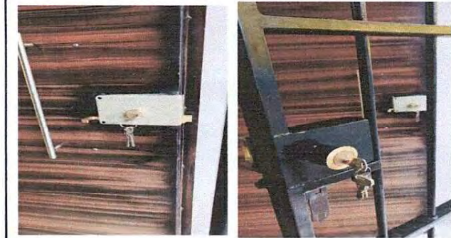
Foto 4: Porton y reja con chapas nuevas, corregido el problema de arrastre del porton, lijados y pintados.
