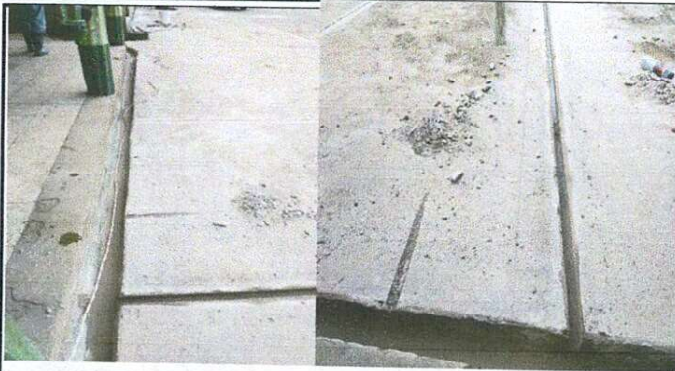
Reparación de planchas de concreto(patio)
