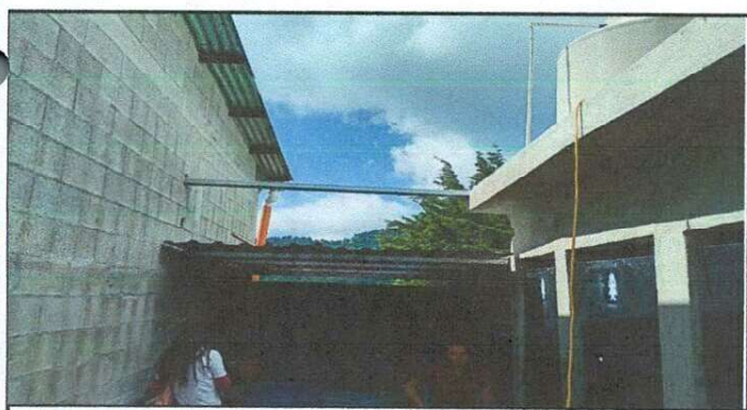
Foto 5: cubierta de lámina en área de baños y estructura de techo
