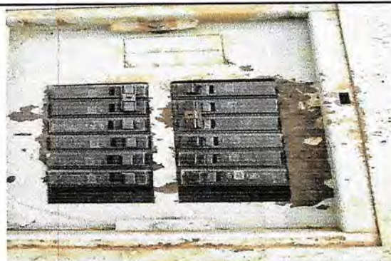
Foto 4: Reparación de sistema eléctrico central con cambio de flopon 20 amperios
