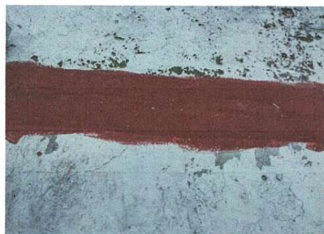
Foto 6: REZANE E IMPERMEABILIZACION DE GRIETA DE MOVIMIENTO
