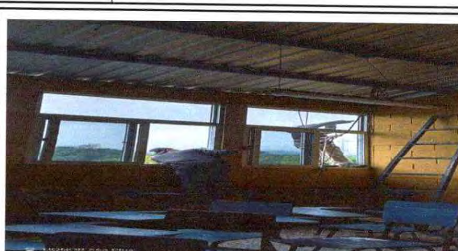
Foto 4: Fabricacion e instalacion de balcones de hierro en ventana con medidas de 1.29 mts de alto por 1.85 metros de ancho color negro.
