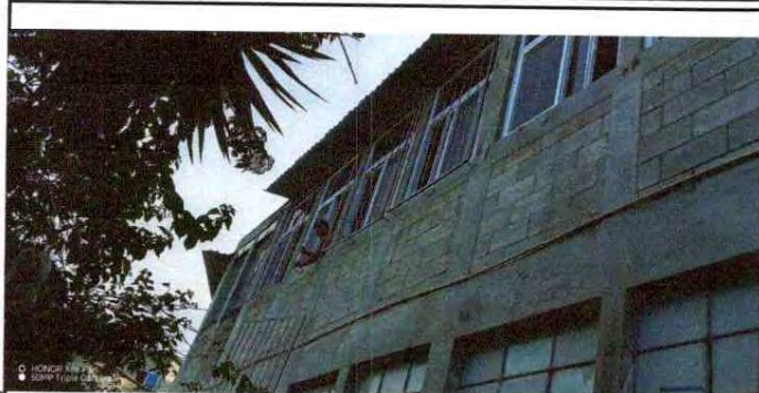
Foto 4: Fabricación e instalación de balcones de hierro en ventana con medidas de 1.29 mts de alto por 1.85 metros de ancho color negro.
