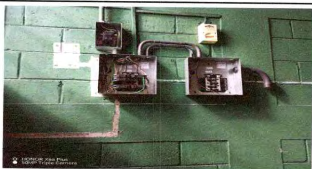
Foto 6: Sustitución de tablero y flipones ( un tablero 2 polos y uno de 8 polos)
