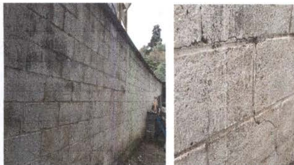
Foto 7: Pared atrás de la Escuela Presenta socavamiento en cimiento y se esta rajando en varias áreas. . (colinda con barranco terreno de un vecino)
