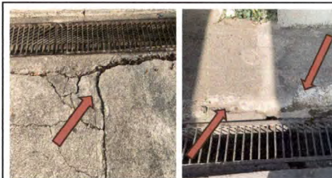
Foto 7 y 8: 8. CUNETA DE CONCRETO 8.1 Reparación de cuneta de concreto
