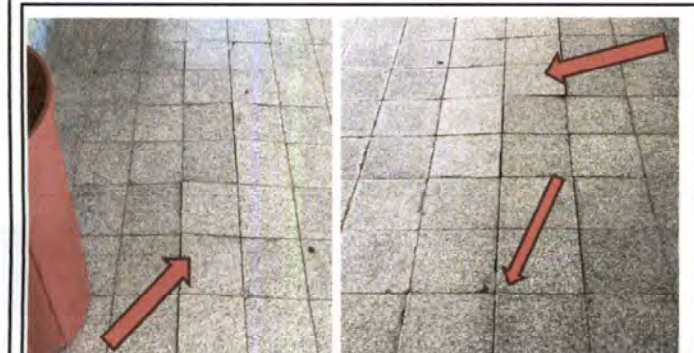
Foto 5 y 6: 6. PISO 6.1 Reparación de piso de torta de concreto de pasillo primer nivel 6.7 Sustitución de piso de granito de pasillo de primer nivel
