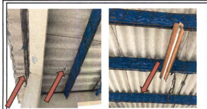
Foto 1 y 2: 1. CUBIERTA DE LÁMINA 1.1 Sustitución de lámina duralita por lámina troquelada de aluzinc calibre 26 1.2 Sustitución de capote para lámina troquelada (techo de gradas)
