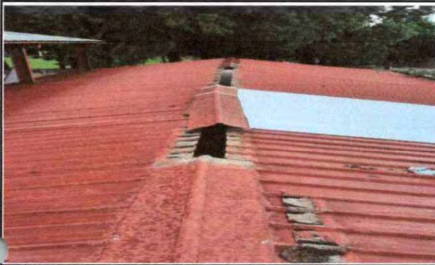
Foto 7. Sustitución de laminas .
