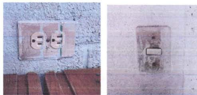
Sustitución de tomacorrientes dobles y apagadores simples por mixtos
