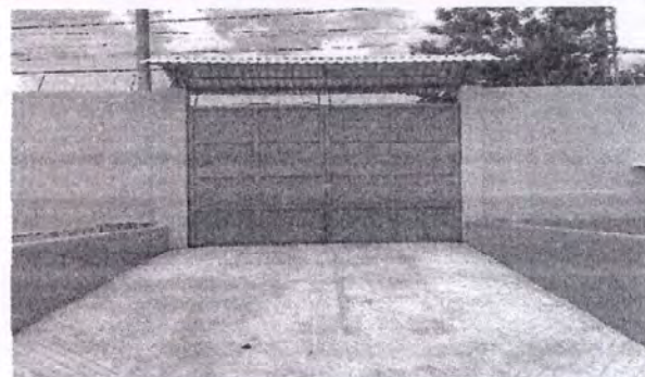
Foto 8: Fabricación e instalación de visera a dos aguas de 5.30 por 3 mts.
