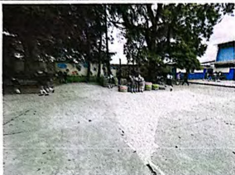
Foto 7: Torta de concreto fundida para nivelar patio de juegos.
