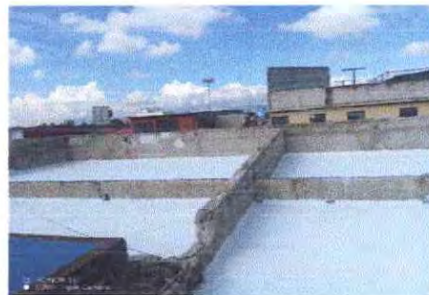
Foto 6: Limpieza y aplicación de impermeabilizante a losa de aulas de escuela 338 metros cuadrados
