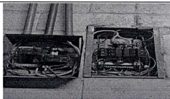
Foto 6: Sustitución de flipones (8 y 12 flipones)
