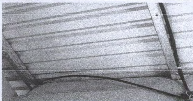
Foto 13: 17.12 Sustitución de ducto eléctrico + accesorios en dirección
