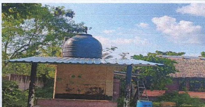
Foto 9: 18.3 Sustitucion de deposito de agua 1700 lt.
