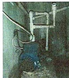
Foto 11: REPACION Y MANTENIMIENTO DE CISTERNAS Y DEPOSITO DE AGUA. 18.3 Sustitución de bomba de agua.
