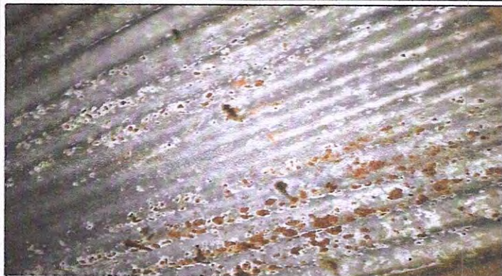
Foto1: 1 CUBIERTA DE LÁMINA: 1.1 Sustitucion de lámina por lámina troquelada aluzinc calibre 26
