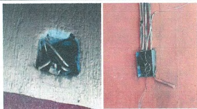
Foto 3: 17. REPARACIÓN DE SISTEMA ELÉCTRICO 17.8 sustitución de tomacorrientes dobles 17.9 sustitución de flipones. 17.10 Sustitución de tablero de flipones.
