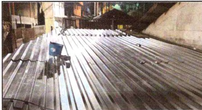
Foto 3: Instalación de lámina troquelada, área exterior de cocina
