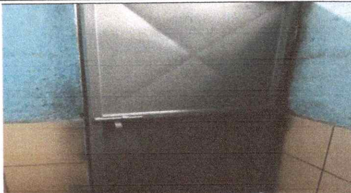
Foto 2: Mantenimiento a estructura, (lijado, cambio de tubo, cepillado, sujeciones, aplicación de pintura)
