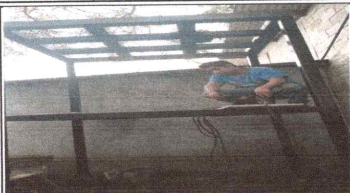
Foto 1: Instalación de estructura portante de metal
