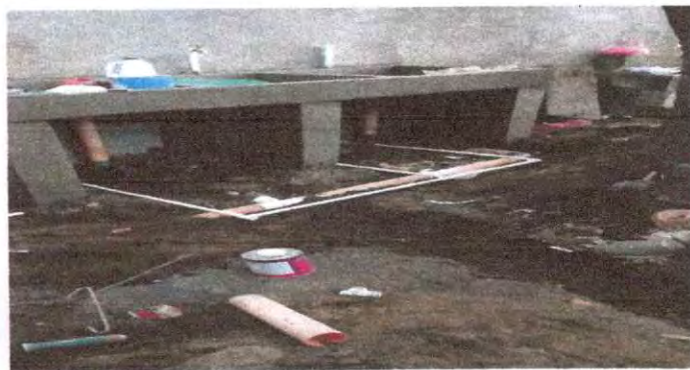
Foto 4: Instalación de tubería para agua potable
